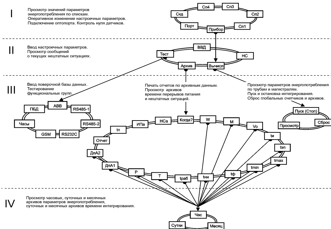
Рисунок 5.1 – Структура меню
